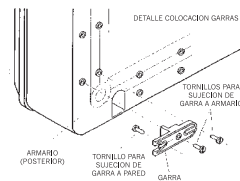
Tipos de fijación a pared
