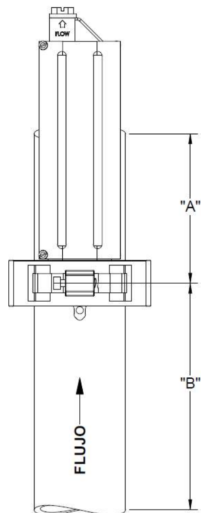
MONTAJE VERTICAL
