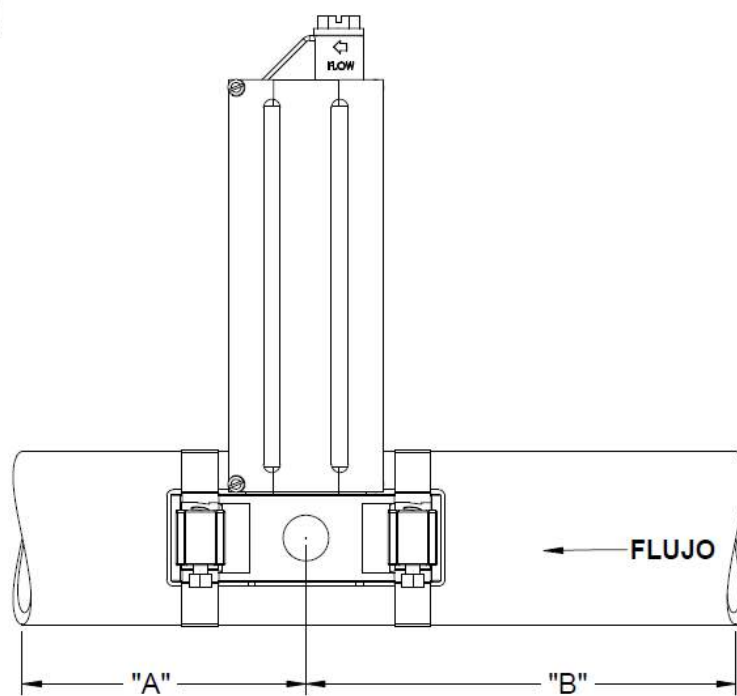
MONTAJE LATERAL
